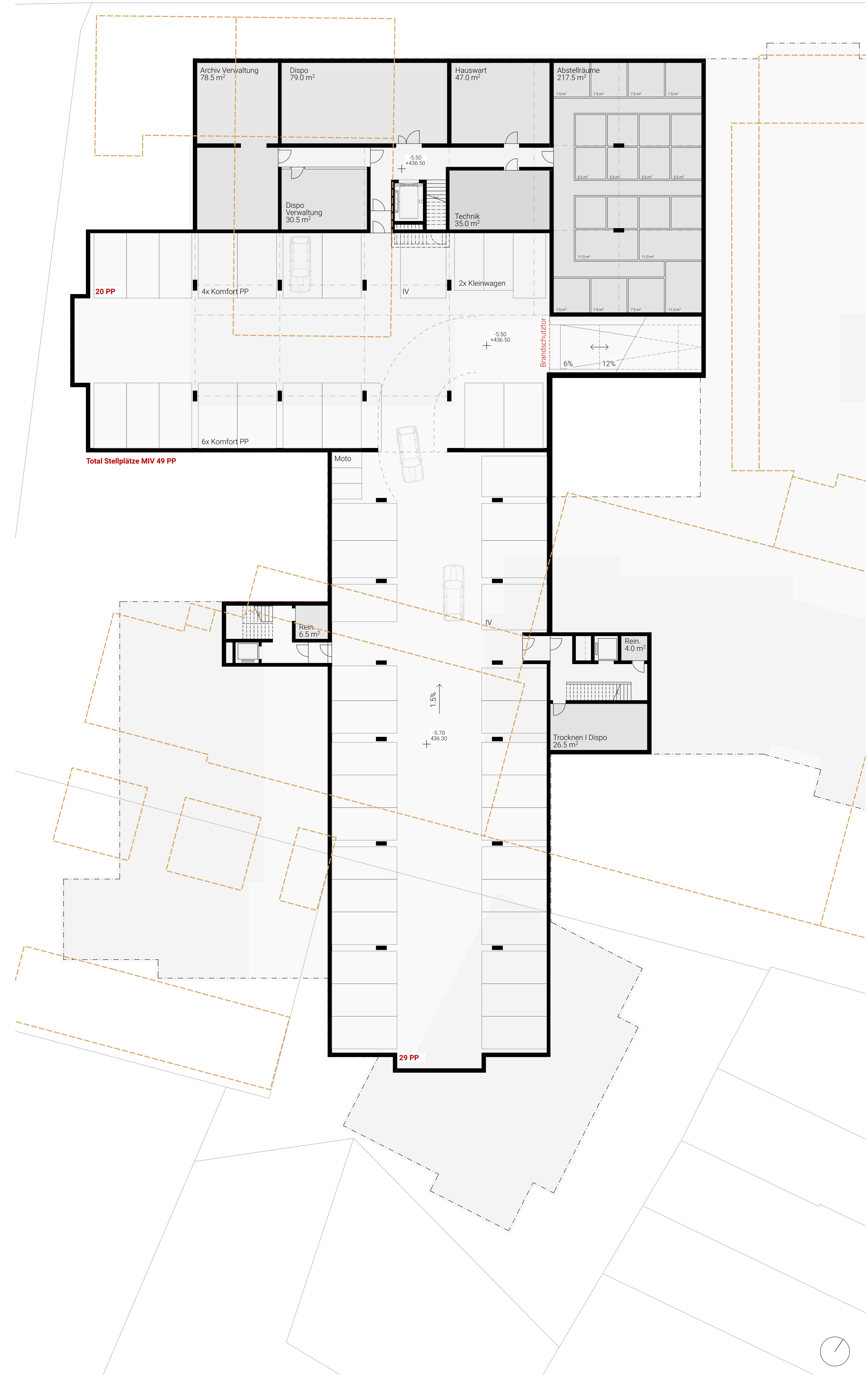
2. Untergeschoss | 1:200
